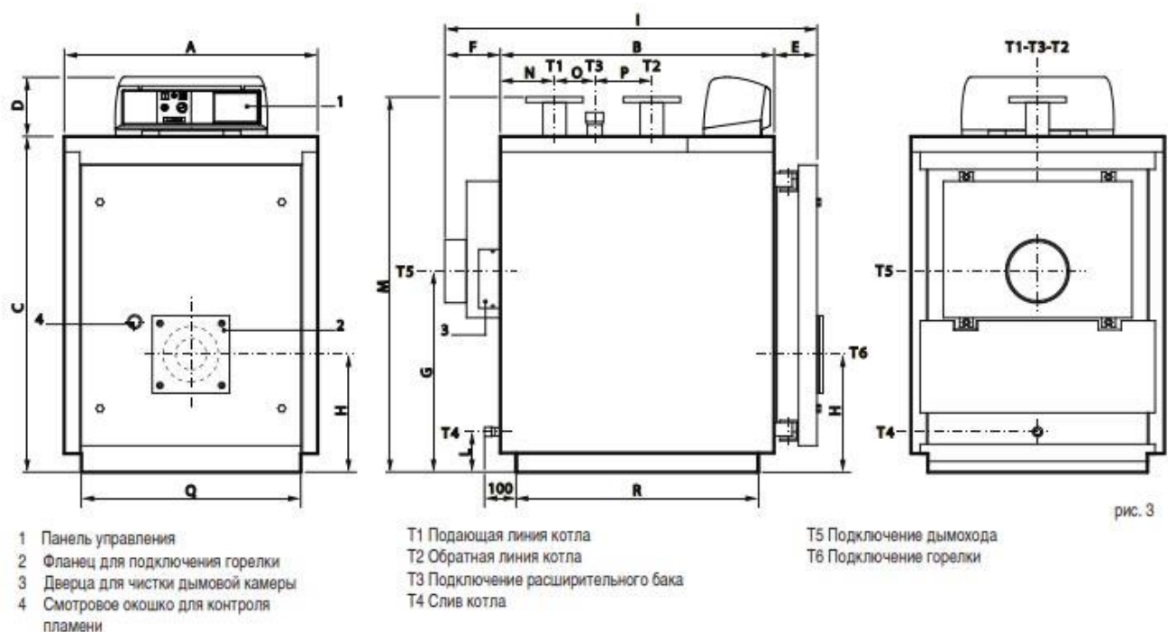
Рисунок 2.1 – Котел Uical ELLPREX 970
