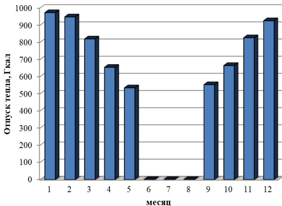
Рисунок 1.2 – Оптимальный температурный график отпуски тепловой энергии для поселковой котельной Томинского сельского поселения
