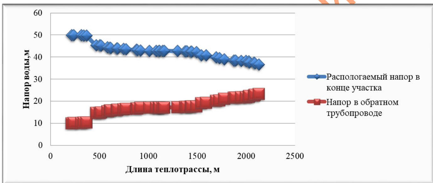
Рисунок 2.4 – Пьезометрический график тепловой сети поселковой котельной п. Томинский по магистральному выводу
