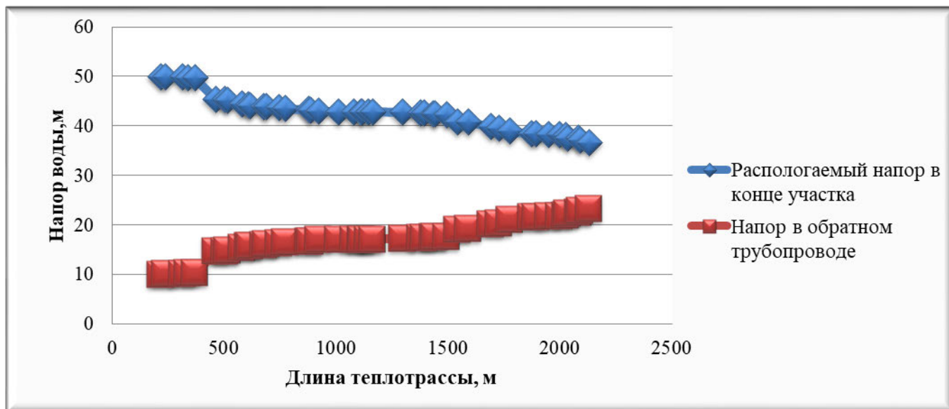
Рисунок 2.5 – Пьезометрический график тепловой сети поселковой котельной п. Томинский по магистральному выводу
